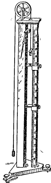
Рис. 32. Машина Атвуда.
