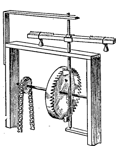
Рис. 24. Регулятор старинных часов — «биянец».
