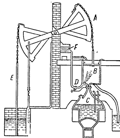
Рис. 35. Машина Ньюкомена.
