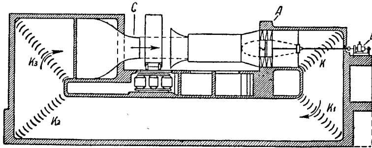
Рис. 53. Аэродинамическая труба,
