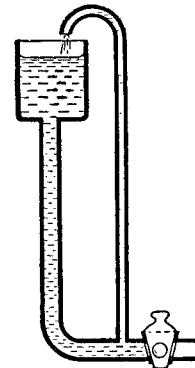
Рис. 51. Осуществление гидравлического удара на опыте.
