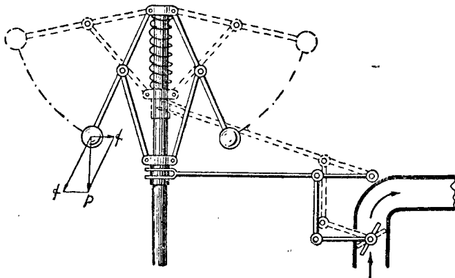
Рис. 28. Центробежный регулятор.
