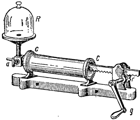
Рис. 21. Воздушный насос Отто Герике.
