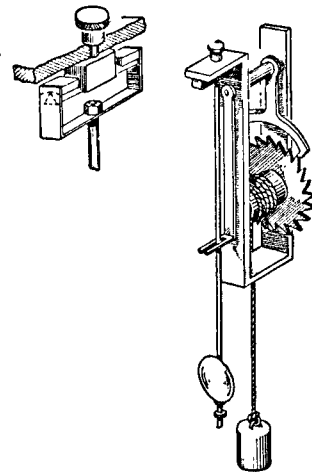
Рис. 25. Регулятор часов, созданный Гюйгенсом.
