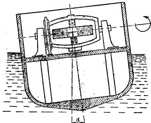
Рис. 46. Успокоитель качки судов.
