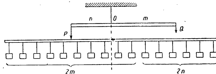
Рис. 6. К доказательству закона рычага.
