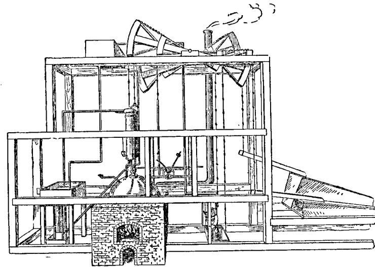
Рис. 36. Машина Ползунова.
