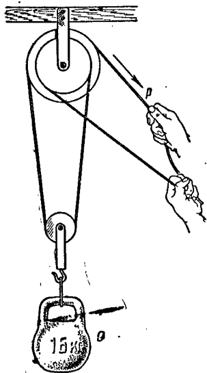
Рис. 18. Дифференциальный полиспаст.
