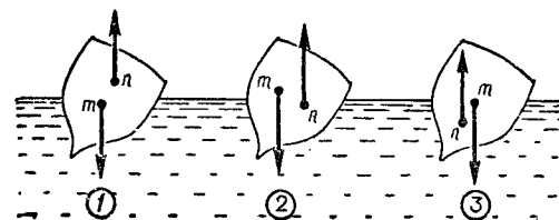
Рис. 14. Равновесие судна.
