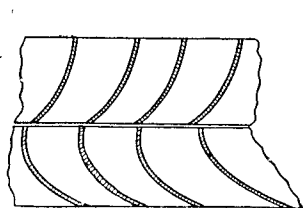
Рис. 49. Направляющее и рабочее колеса реактивной турбины Жонваля.
