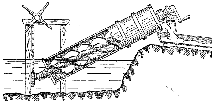
Рис. 2. Архимедов винт.
