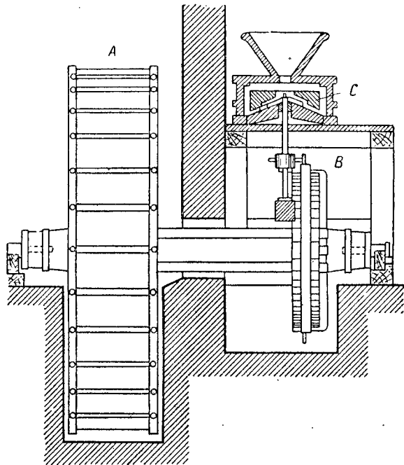
Рис. 3. Римская водяная мельница.
