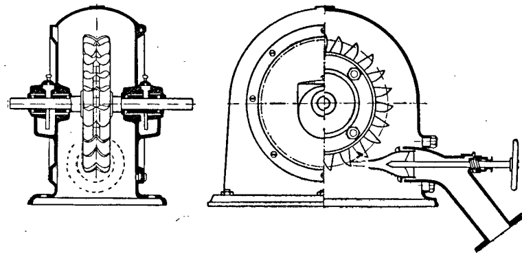
Рис. 48. Турбина Пельтона.
